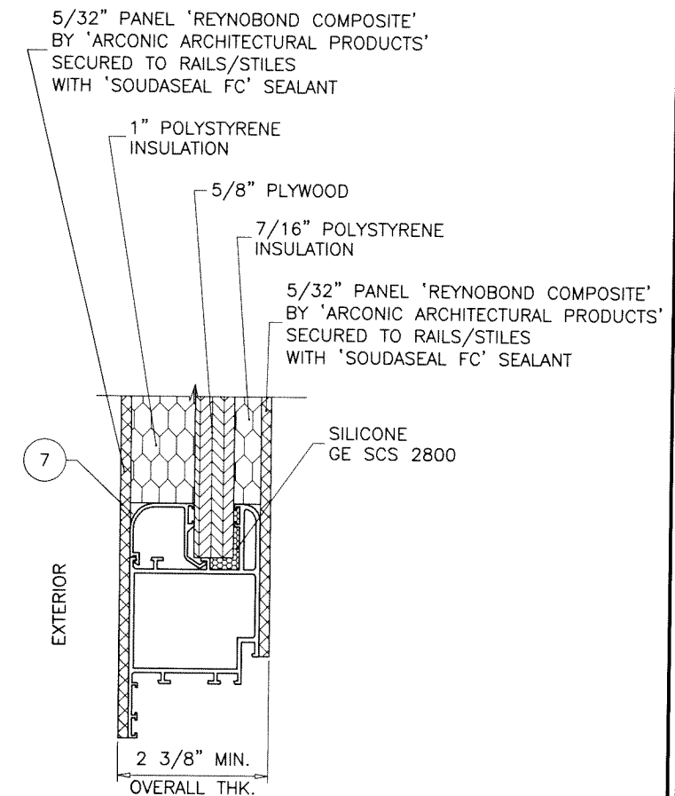
OPAQUE DOOR
