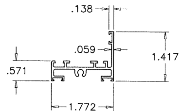
1A FRAME SILL
